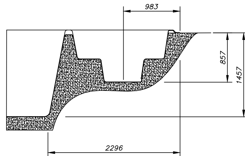
CORTE-BB ESC.:1:40
