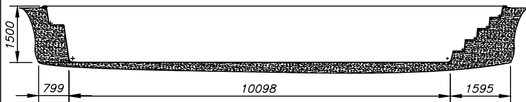
CORTE-AA ESC.:1:75
